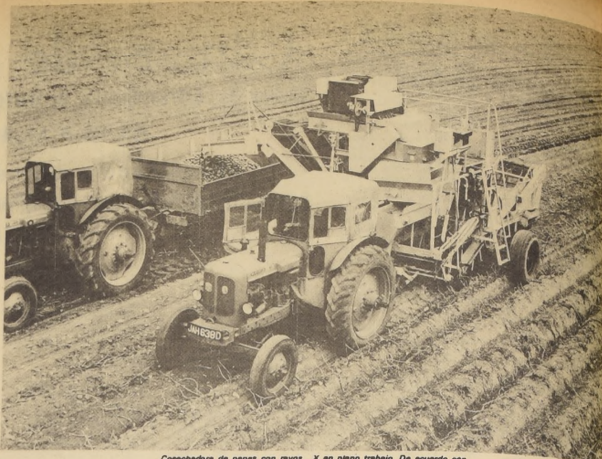
Cosechadora de papas con rayos X en pleno trabajo. De acuerdo con las condiciones, la separación de las papas por un lado y las piedras y terrones por otro puede alcanzar un rendimiento del 95 por ciento.
