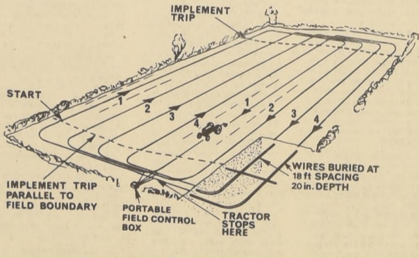
Diagrama ilustrativo del sencillo sistema de "red de cables" para el tractor sin conductor. Si se realiza un trabajo de drenaje la red puede ser sepultada a mayor profundidad, por un costo ligeramente superior. 1) Punto de partida; 2) Límite de recorrido del implemento; 3) Cables sepultados a intervalos de 5,49 metros y 0,50 metros de profundidad; 4) Punto de detención del tractor; 5) Caja portátil de control de campo; 6) El límite de recorrido del implemento es paralelo al límite del campo.
