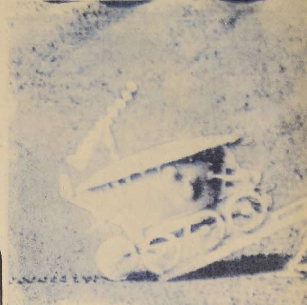
El Lunajod 1 que aterrizó el lunes en la Luna, en el Mar de las Lluvias, es el primer explorador automático concebido por el hombre para desentrañar los misterios del satélite natural de la Tierra. El artefacto, semejante a un gran samovar de plata, se desplaza sobre ocho ruedas y está dirigido por control remoto desde la Tierra. A su bordo lleva un cargamento científico que comprende cámaras de televisión que han transmitido clarísimas imágenes de la luna hasta las pantallas de los televisores soviéticos. También está dotado de un reflector de rayos Láser y un equipo de radio capaz de recibir señales. (Foto UPI).
