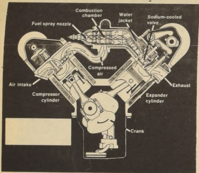
Diagrama del nuevo motor Warren, limpio y económico en su uso
