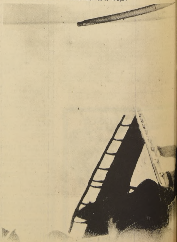
"Lunokod-1" en la plataforma de alunizaje de la estación "Luna-17" momentos antes de descender a la superficie de la Luna. Foto tomada por el televisor de a bordo de "Lunokod-1". Se ve el paisaje lunar delante del aparato, la rampa de descenso de "Luna-17" desplegada y la antena de varillas de "Lunokod". (FOTO TASS-APN).
