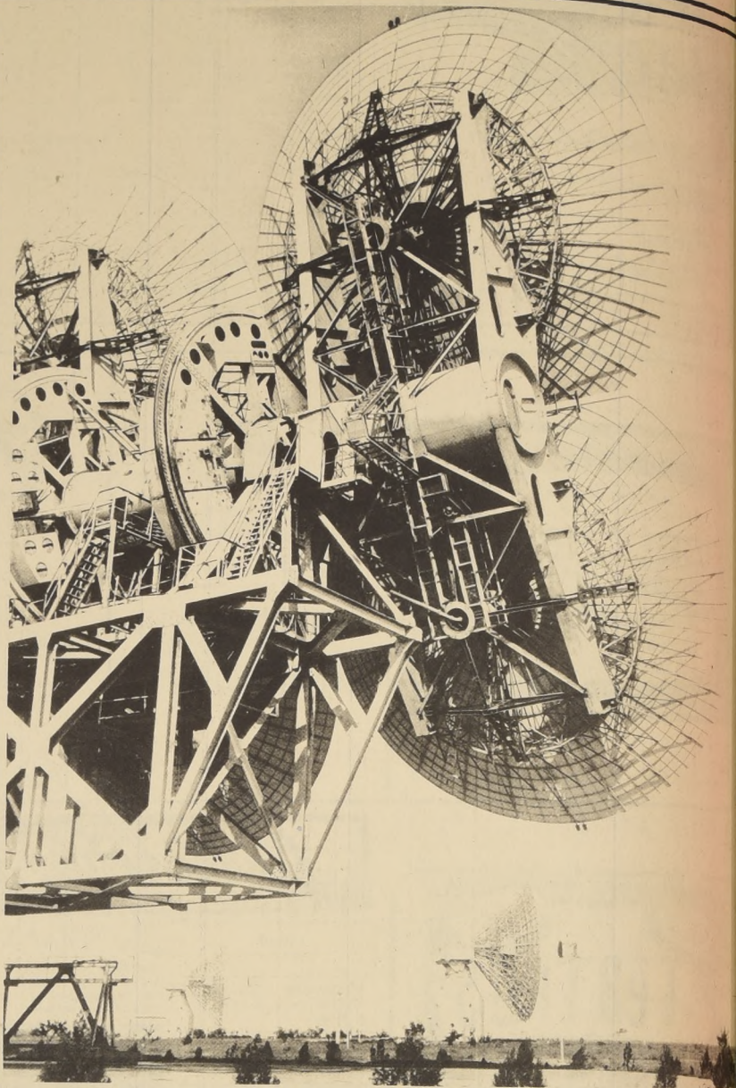
Puesto de telecomunicaciones cósmicas. Desde aquí se mantenían las comunicaciones con las estaciones "Venera-5" y "Venera-6". (FOTO APN).
