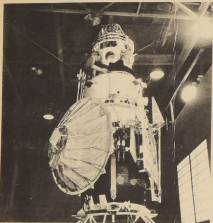
El 18 de octubre de 1967 la estación automática soviética "Venera-4", al cubrir unos 35 millones de kilómetros, se posó suavemente en la superficie de Venus, por primera vez en la historia de astronáutica, y transmitió desde allí valiosísimos datos. En la parte inferior se ve el módulo descendente, el laboratorio científico. (APN).
