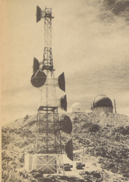
Estación repetidora de Microondas en Cerro Tololo, de la Red Troncal Nacional. Al fondo, el Observatorio Astronómico de AURA Inc. ENTEL - CHILE.
