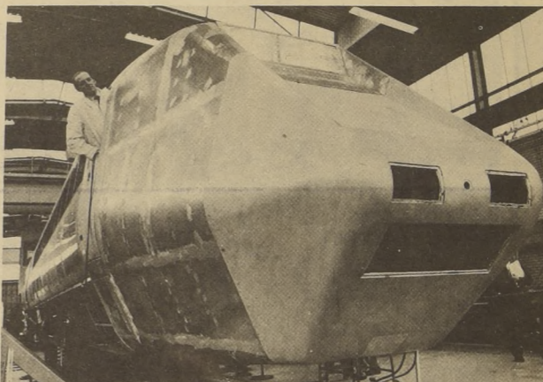
UNO DE LOS CARROS MOTORES del tren de pasajeros APT—E de los Ferrocarriles Británicos visto en etapa de construcción. De casi 33 metros de largo, cada carro contiene cuatro motores Leyland de turbina a gas, para fines de tracción, mientras que un quinto motor suministra calor, aire acondicionado, iluminación y equipo de control.
