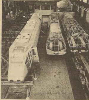
VISTA GENERAL DEL LABORATORIO de Proyectos Avanzados de Ferrocarriles Británicos, que muestra el carro motor de nariz de bala del tren de pasajeros APT—E (izquierda) y dos POP (Energía sin-Energía), tren compuesto por un equipo rudimentario de dos carros de espaciada armazón en su estructura, para ser usados en desarrollo de suspensión.
