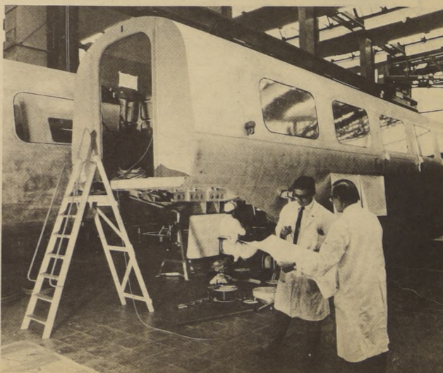
LOS DOS CARROS QUE FORMARÁN parte del tren APT—E han sido sometidos ya a una serie de presiones y pruebas. Se les está acomodando para incorporarles los instrumentos y el equipo requerido en las carreras de prueba más avanzadas este año.
