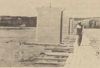
Puente Itata, en Coelemu, en construcción, visitado por el Ministro Pascual Barraza.
