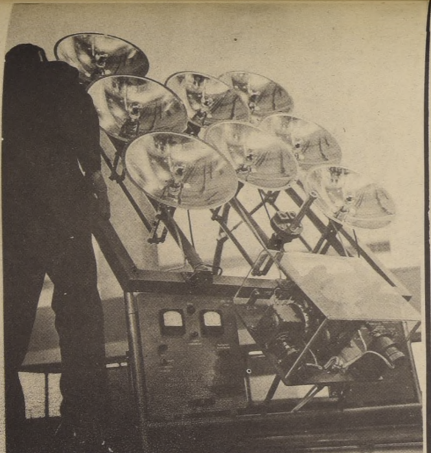
Montaje de un modelo experimental de termo-elektrogenerador solar de semiconductores, ideado por científicos del Instituto de Investigación Energética G. Krzhizhanovski, de Moscú.
