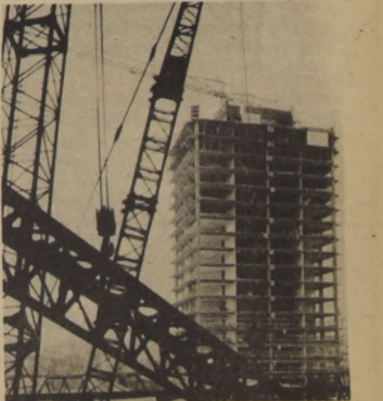
La UNCTAD III fue el gran desafío para Chile. En el grabado, el edificio en su etapa de acelerada construcción. La obra estuvo terminada dentro de los plazos fijados, gracias al esfuerzo de profesionales, técnicos y trabajadores.
