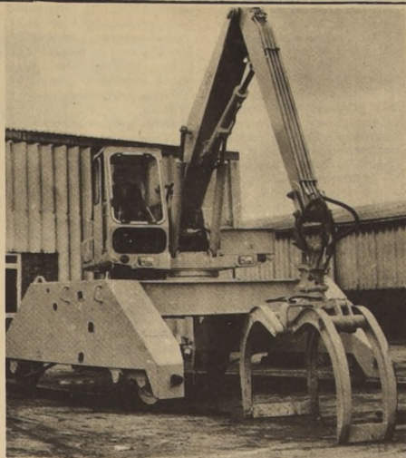
MAQUINARIA BRITANICA PARA CHILE. Seis máquinas similares a ésta, fueron adquiridas por la Empresa Chilena CELCO, para la movilización de troncos en la nueva planta productora de pulpa de madera y celulosa, que se levanta en Constitución, en la Provincia de Maule. Las máquinas fueron adaptadas especialmente para su utilización en dicha planta y están provistas de ganchos. Son de autopropulsión. Tres van montadas sobre rieles y el resto sobre ruedas neumáticas.
