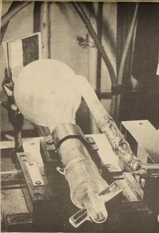
REACTOR DE CUARZO para obtener cristales filiformes de diamante.
