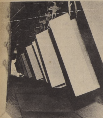
Piezas de califontes Junkers, transportadas por la correía sin fin, a lo largo del túnel de secado.
