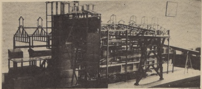
CON UN NUEVO HORNO REVERBERO contará, a partir del mes de mayo, la Fundición de Caletones del Mineral "El Teniente". La nueva obra permitirá aumentar la actual producción de cobre fino en 200 toneladas, con equivalencia de US$ 200 mil por día. Vale decir, que la Fundición quedará en condiciones de entregar al país unas 900 toneladas de cobre al día. El nuevo horno fue ejecutado y diseñado enteramente por trabajadores chilenos y, por primera vez, no ha sido necesario pagar a otros países por licencias o patentes extranjeras. También se han aprovechado todos los recursos nacionales con respecto a materiales y equipos. Ello permitió mantener el gasto de divisas en apenas un 10% de la inversión total, que alcanza a 120 millones de escudos. El desafío del moderno horno reverbero, que concentra las técnicas más avanzadas sobre fundición, comenzó en el mes de enero del año pasado y en él participaron aproximadamente 300 trabajadores. EN LA FOTO un modelo a escala del horno con que contará la Fundición de Caletones.
