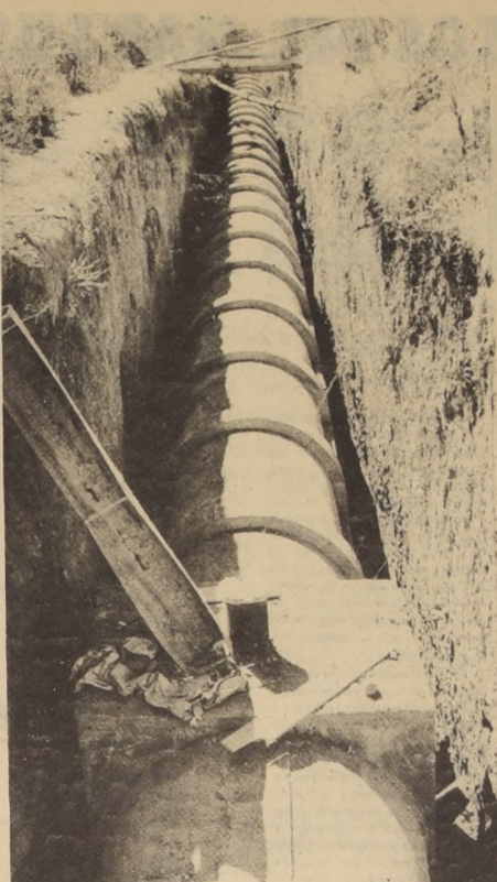
Parte del primer tramo del Tercer Acueducto que pondrá fin a los problemas de abastecimiento de agua potable a diversas comunas periféricas de la provincia de Santiago. La tubería, con un tramo de cerca de dos mil metros, forma parte del sistema que hoy se pondrá en marcha, con asistencia del Presidente Allende.
