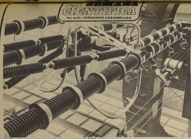
750 mil voltios de tensión enviados a 1.100 kilómetros
